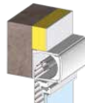
Volet roulant intégré enroulement intérieur
