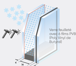
Vitrage 4 ITR/14 argon/44.6 (SP510) Verre sécurité renforcée classé P5A selon la norme EN 356 : protection contre l'effraction. Coefficient Ug 1.1
