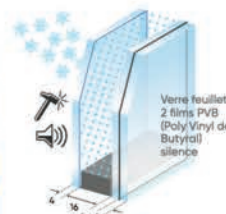
Vitrage 4 ITR/16 argon/44.2 Silence Verre acoustique et sécurité coefficient Ug 1.1
