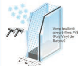
Vitrage 4 ITR/14 argon/44.6 (SP510) Verre sécurité renforcée coefficient Ug 1.1
