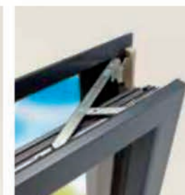
Détail système oscillo-battant
