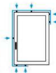
Quincaillerie à renvoi d'angle Chaînage des éléments avec renvoi en partie horizontale. Meilleur maintien du vantail. Optimise la sécurité de la menuiserie. Améliore la compression.
